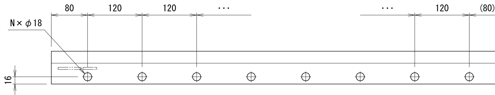
全体図(1:5)
