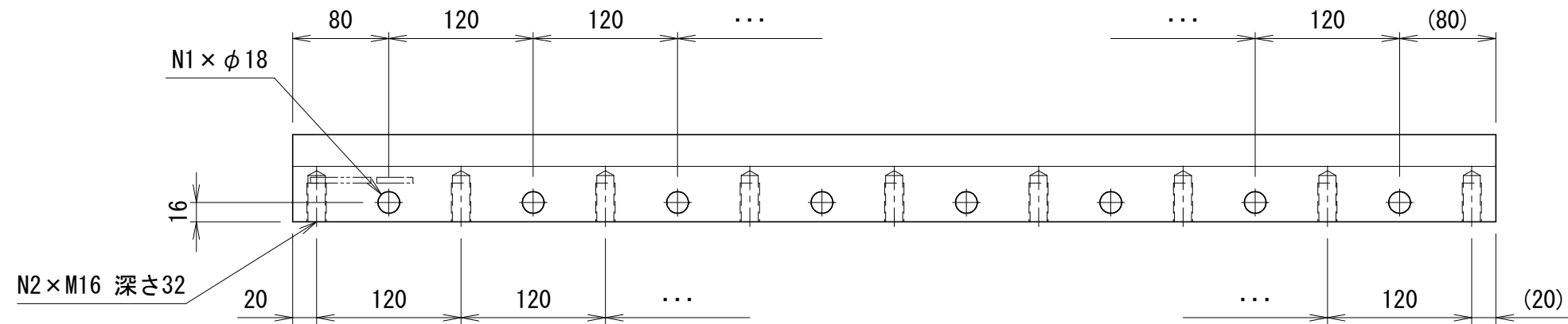
全体図(1:5)
