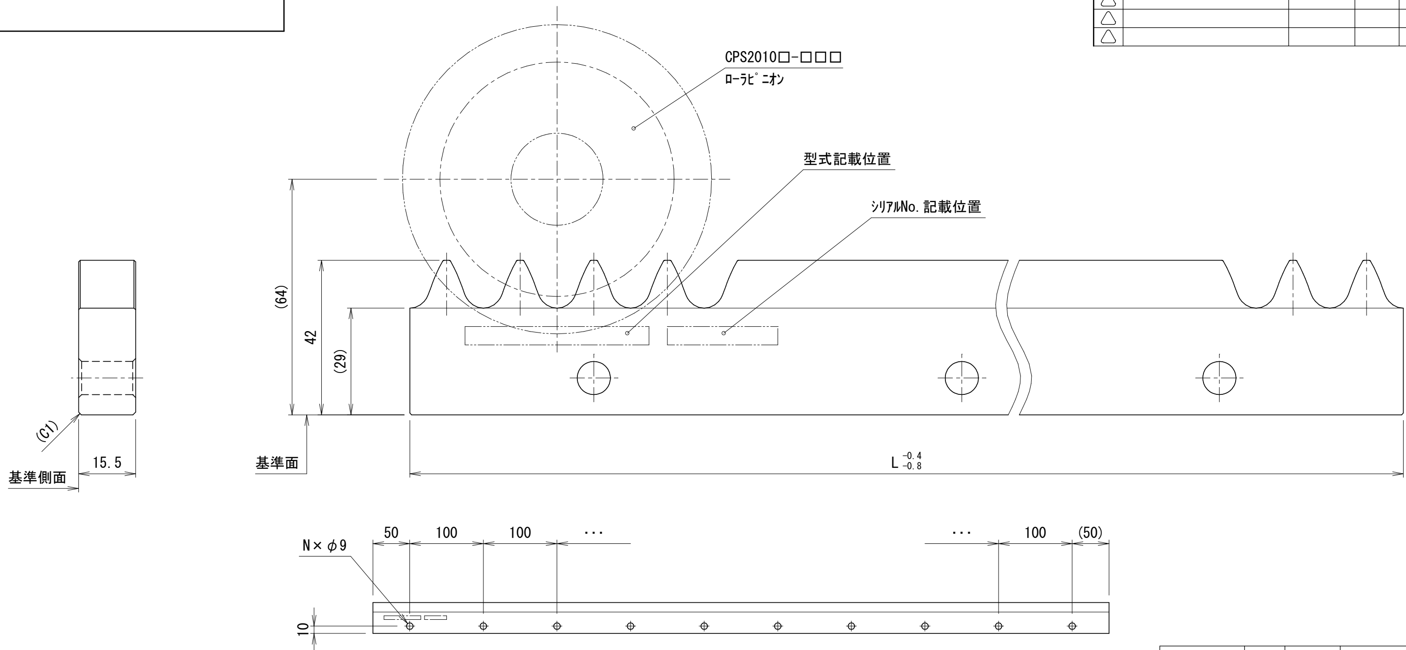
全体図(1:5)
